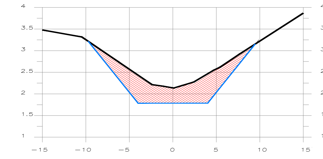
SECCION 0+490
