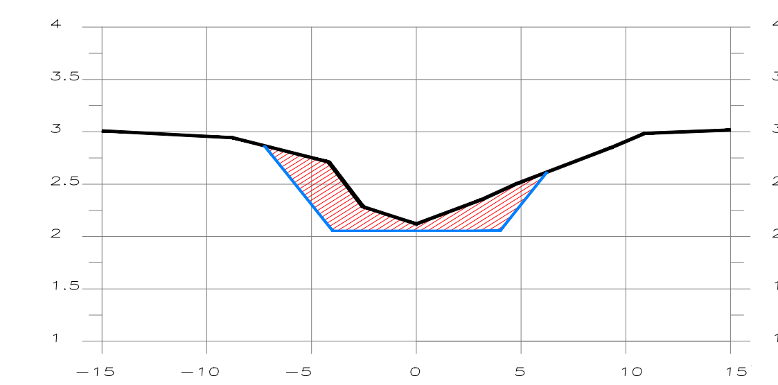
SECCION 0+682.09
