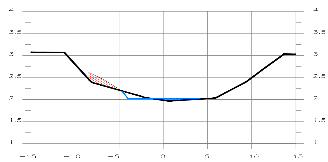
SECCION 0+660
