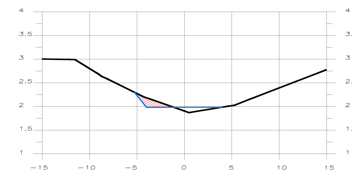
SECCION 0+630
