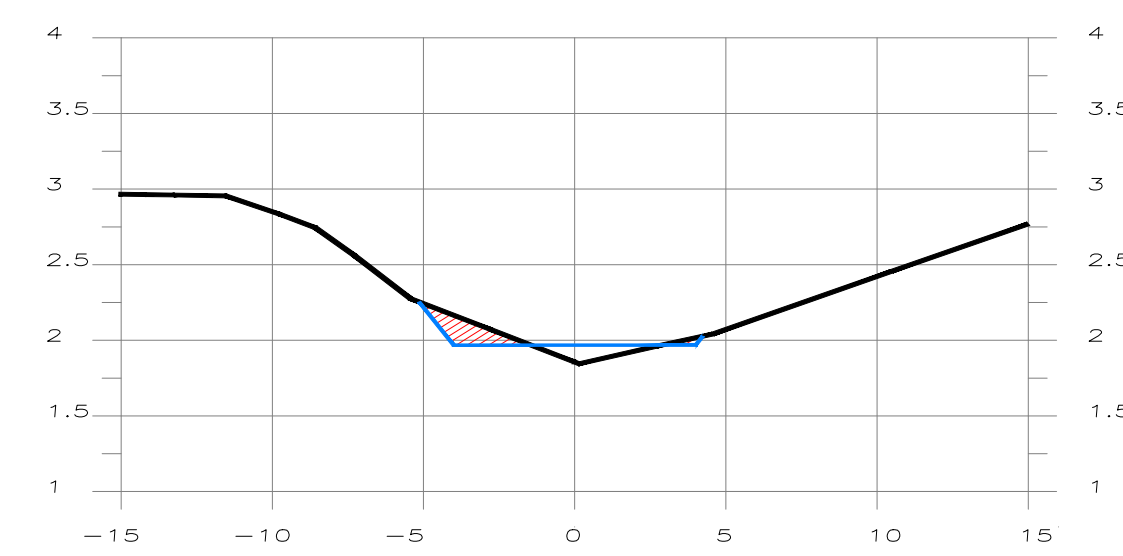
SECCION 0+620
