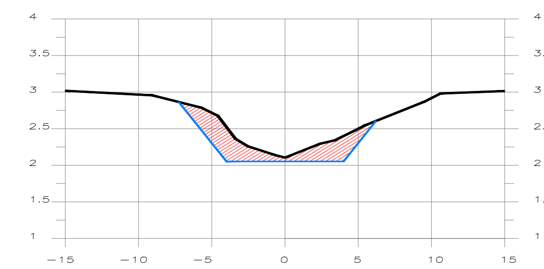
SECCION 0+680
