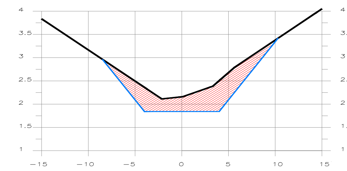
SECCION 0+530
