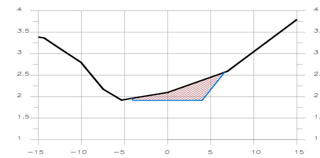
SECCION 0+580
