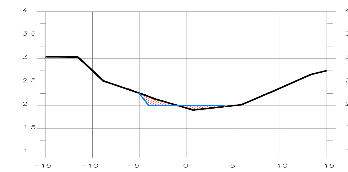
SECCION 0+640
