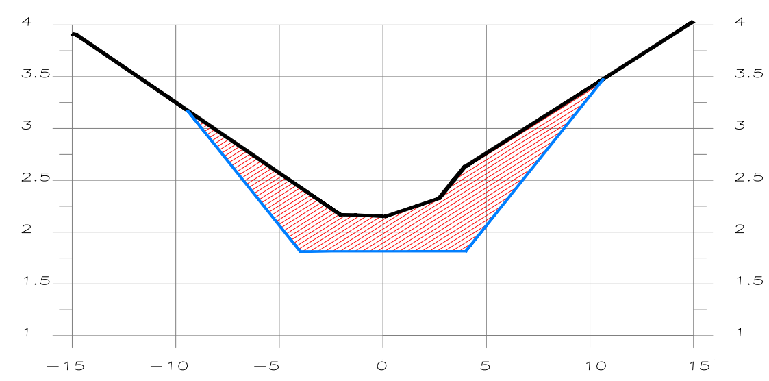
SECCION 0+510
