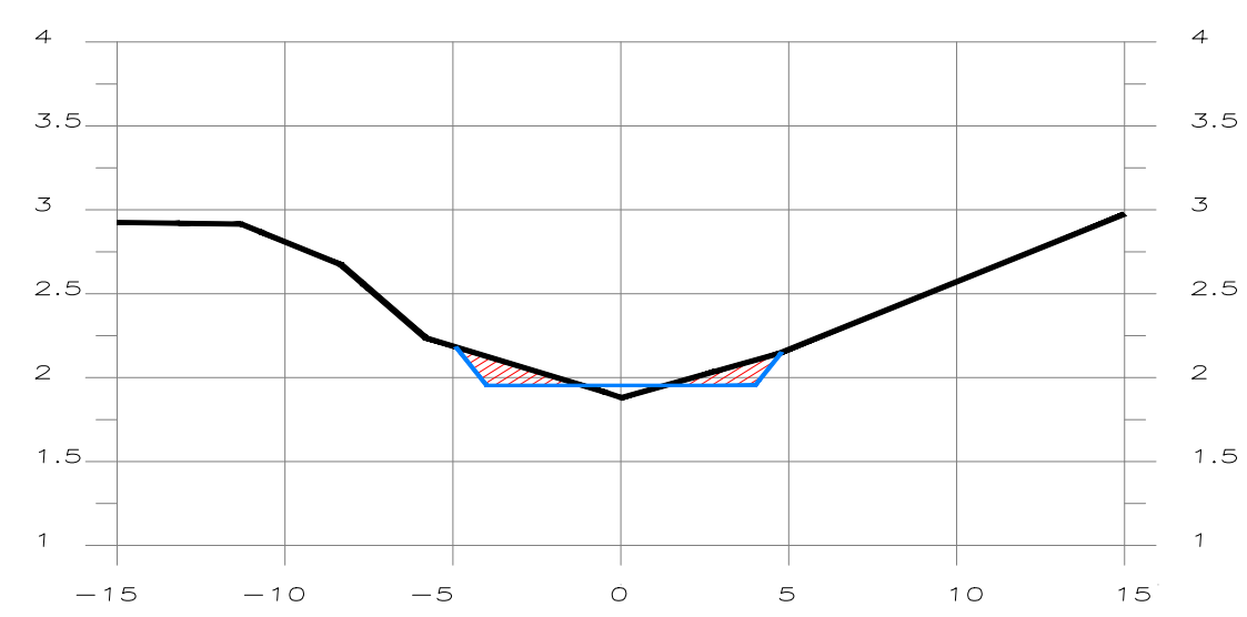
SECCION 0+610
